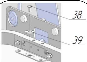
Рис.9.3 Регулировка положения щитов
