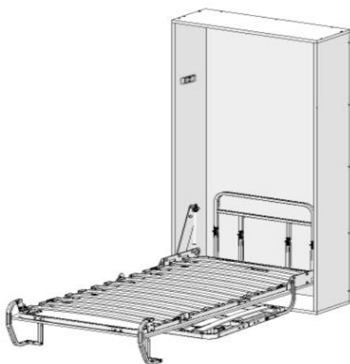
Рис.27.1 Кровать разложена
